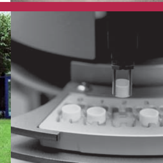
Automatischer Probengeber einer Thermogravimetrie-Massenspektrometrie mit Keramiktieglern
